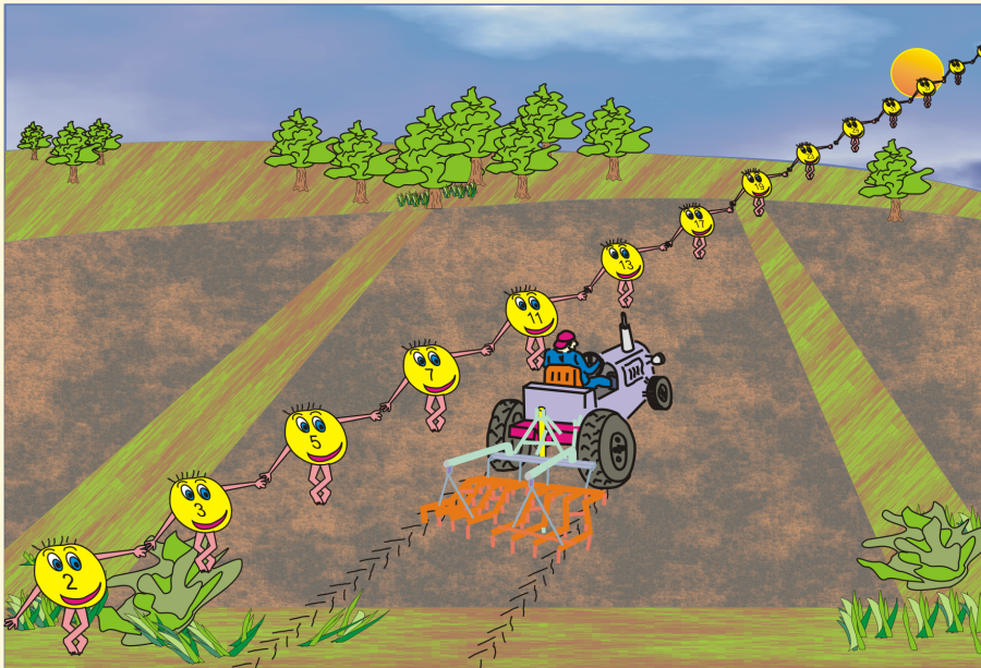
Obr. 2.1 Posloupnost prvočísel roste nade všechny meze.
