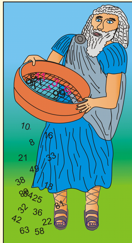
Obr. 2.2 Eratosthenovo síto na prvočísla
