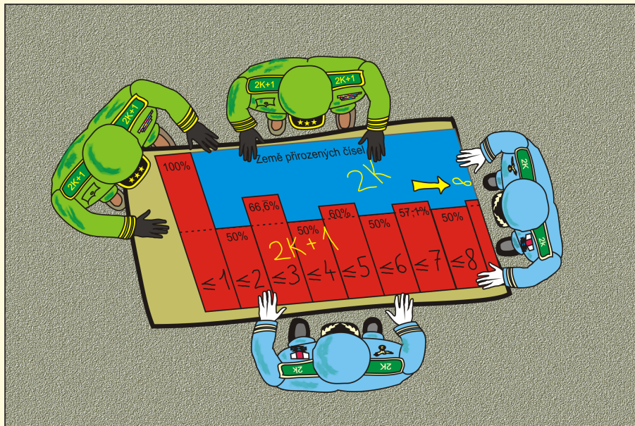
Obr. 3.1 Sudá a lichá čísla si rozdělují množinu přirozených čísel.
