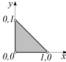
Obr. 5.5 Příklad trojúhelníkového prvku pro sestavení matice tuhosti [K_e]
