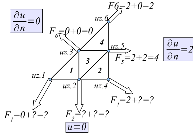
Obr. 5.11 Grafické ztvárnění údajů MKP rovnice
