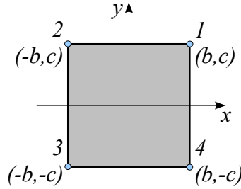
Obr. 5.6 Bilineární obdélníkový prvek
