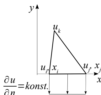
Obr. 5.7 Okrajová podmínka pro hraniční integrál
