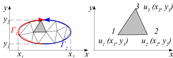
Obr. 5.3 Diskretizace oblasti \Omega na elementy; umístění elementu v souřadnicích x, y
