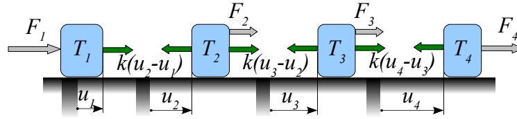
Obr. 4.4 Uvolnění soustavy čtyř těles spojených pružnými členy
