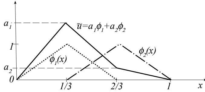
Obr. 2.2 Přibližné řešení \tilde{u}(x) pomocí funkcí \phi_1(x) a \phi_2(x)
