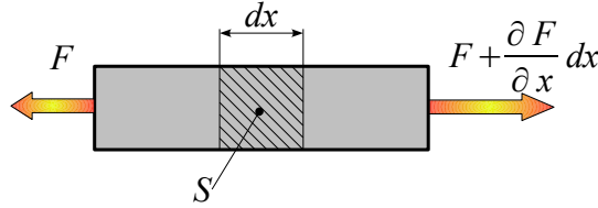
Obr. 3.1 Uvolnění elementu dx prutového prvku
