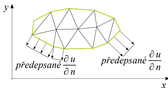
Obr. 5.7 Okrajová podmínka pro hraniční integrál
