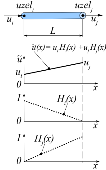
Obr. 3.2 Grafické znázornění funkcí tvaru H(x) a jejich významu ve vztahu (3.13)
