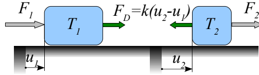
Obr. 4.2 Dvě tělesa spojená pružným členem
