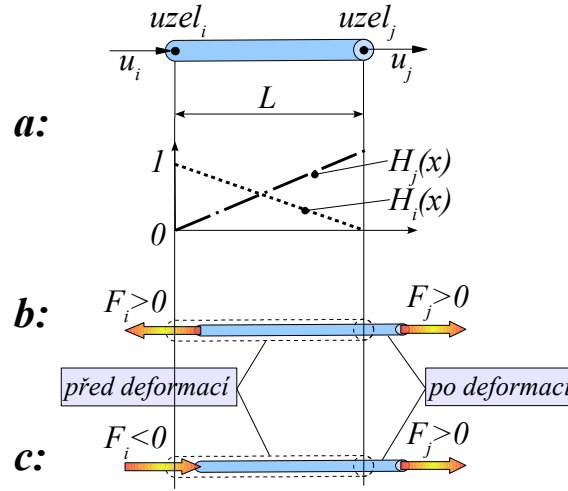
Obr. 3.3 Grafické znázornění von Neumannových okrajových podmínek a jejich fyzikálního významu ve vztahu (3.28)
