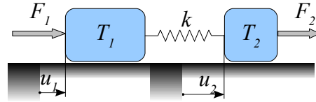
Obr. 4.1 Dvě tělesa spojená pružným členem
