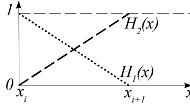
Obr. 2.5 Lineární funkce tvaru H_1(x), H_2(x)
