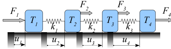
Obr. 4.3 Soustava čtyř těles spojených pružnými členy
