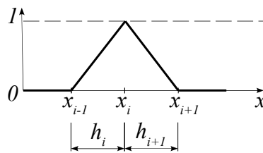
Obr. 2.1 Po částech lineární funkce
