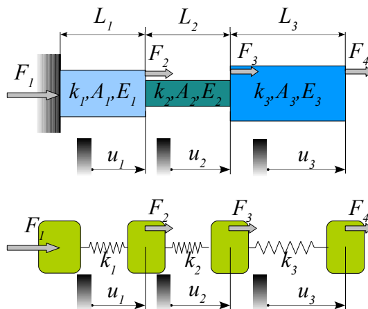
Obr. 4.5 Axiálně namáhaná osazená tyč
