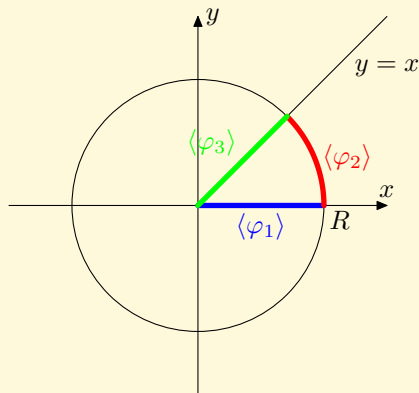
Obr. 3.3: k = \langle \varphi_1 \rangle \cup \langle \varphi_2 \rangle \cup \langle \varphi_3 \rangle z příkladu 3.11c)
