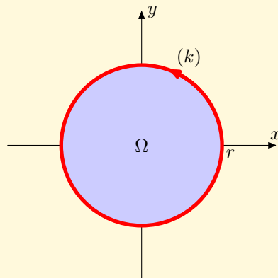
Obr. 3.13: Ilustrace k příkladu 3.29d)
