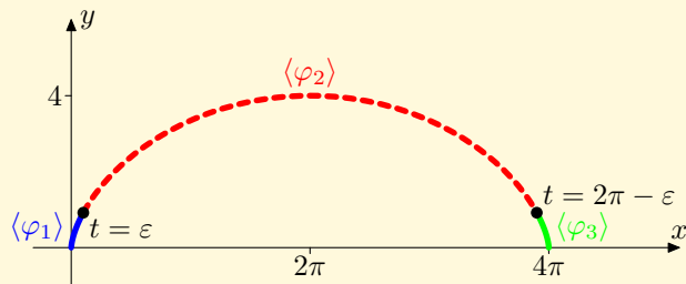
Obr. 3.4: \langle \varphi \rangle = \langle \varphi_1 \rangle \cup \langle \varphi_2 \rangle \cup \langle \varphi_3 \rangle z příkladu 3.11d)
