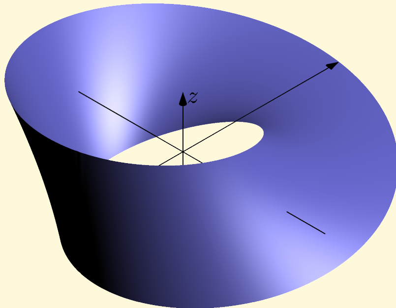
Obr. 6.1: Möbiův list
