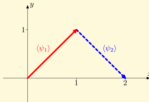
Obr. 3.6: \langle \varphi \rangle = \langle \psi_1 \rangle \cup \langle \psi_2 \rangle z příkladu 3.17 b)
