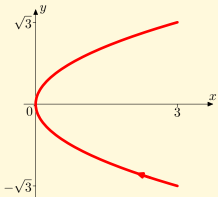
Obr. 3.7: (k) z příkladu 3.21 a)
