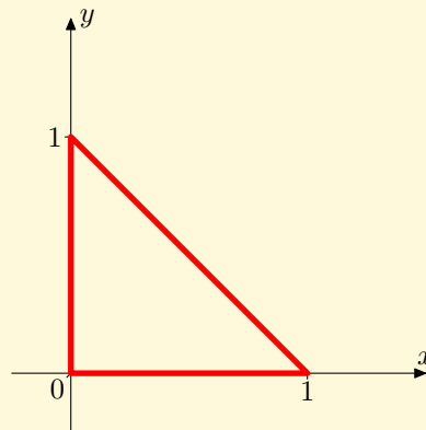
Obr. 3.2: k z příkladu 3.11b)
