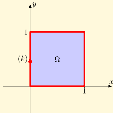
Obr. 3.12: Ilustrace k příkladu 3.29c)
