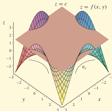
Obr. 1.7: Vrstevnice
