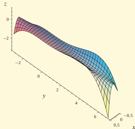
c) (x, y) \in \langle -0,5; 0,5 \rangle \times \langle -4; 7 \rangle
