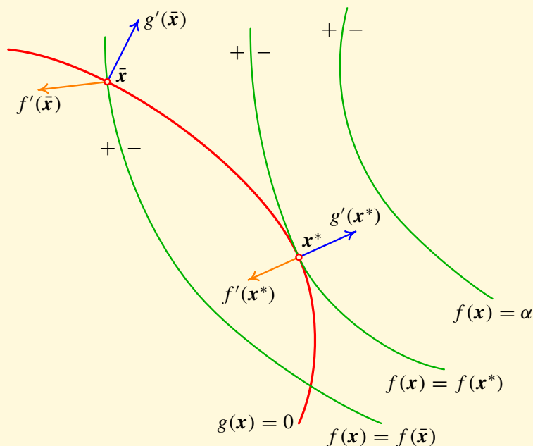
Obr. 8.1: Nutná podmínka existence lokálního extrému v klasické úloze na vázaný extrém
