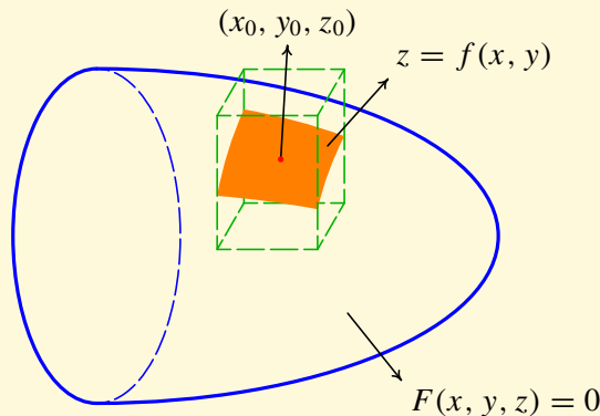
Obr. 7.5: Funkce dvou proměnných daná implicitně
