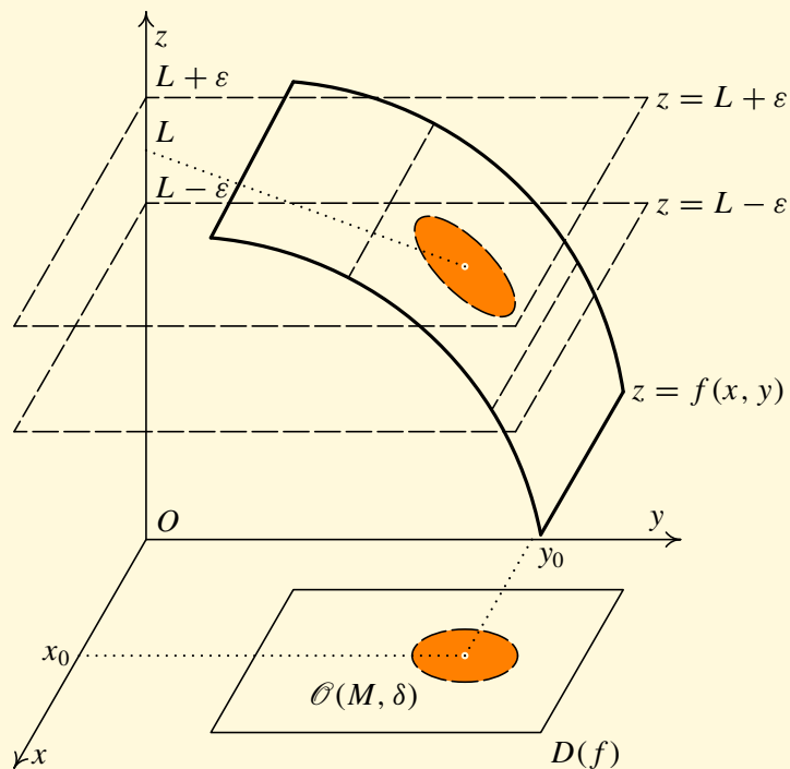
a) Vnitřní bod D(f)
