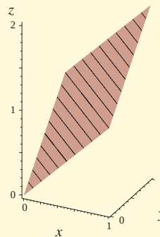
b) k: z = x + y
