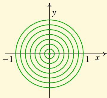
a) Vrstevnice
