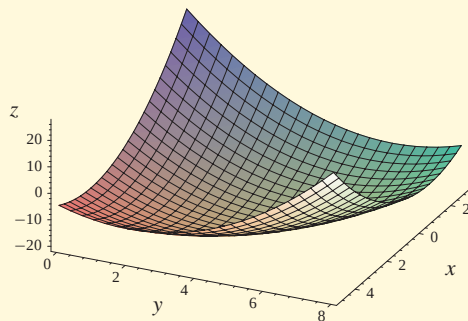
Obr. 5.3: Graf funkce f: z = x^2 + xy + y^2 - 6x - 9y
