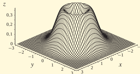
Obr. 5.7: Graf funkce
