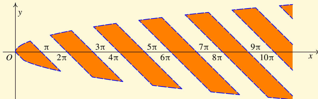
Obr. A.3: Definiční obor funkce z = \frac{\ln \sin(x+y)}{\sqrt{x-y^2}}
