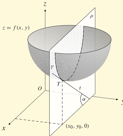
Obr. 2.2: Geometrický význam derivace
