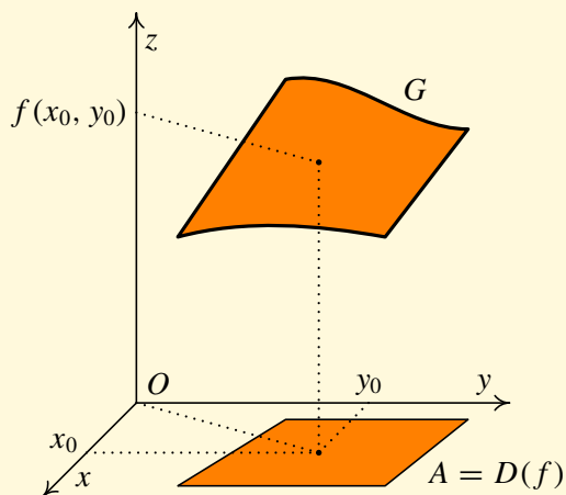
a) G je grafem funkce
