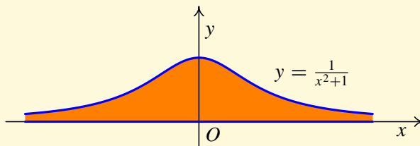
Obr. A.4: Definiční obor funkce z = \arcsin[2y(1 + x^2) - 1]
