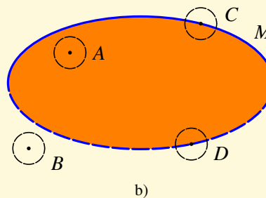
Obr. 1.1: Okolí a klasifikace bodů v rovině
