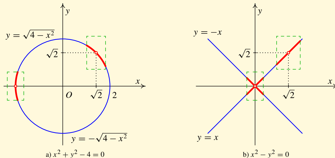
Obr. 7.1: Funkce dané implicitně
