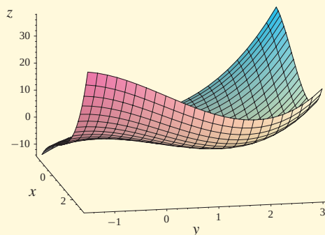
Obr. 5.4: Graf funkce f: z = x^3 + y^3 - 3xy
