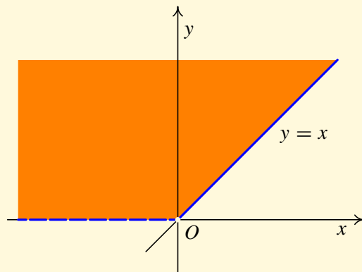
Obr. A.1: Definiční obor funkce f: z = \sqrt{y-x} \cdot \ln(x^2y)
