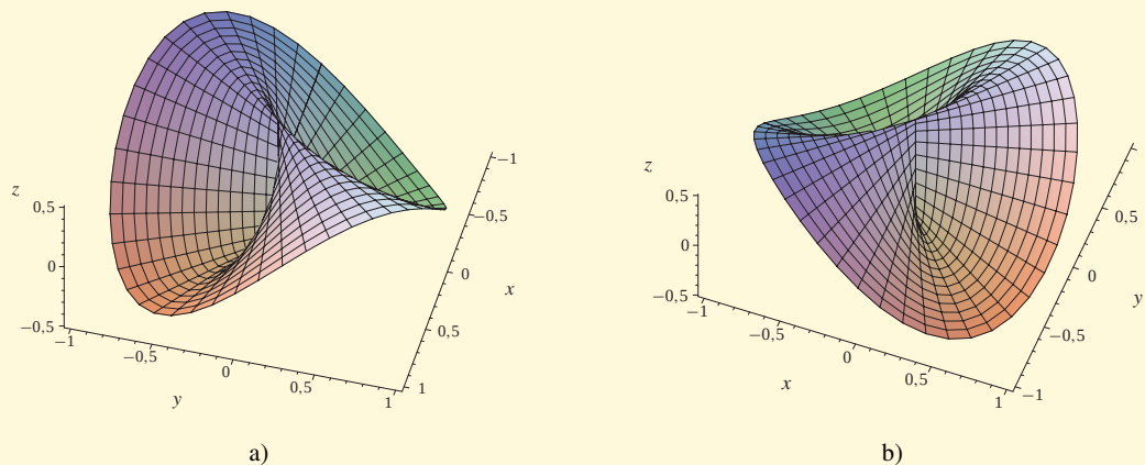
Obr. 1.11: Graf funkce f(x, y) = \frac{xy}{x^2 + y^2}
