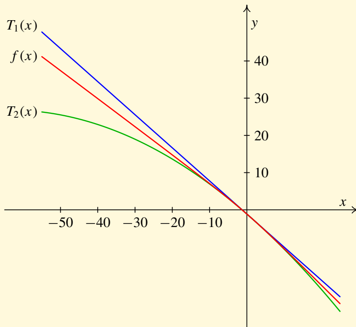
Obr. 7.3: Graf funkce dané implicitně
