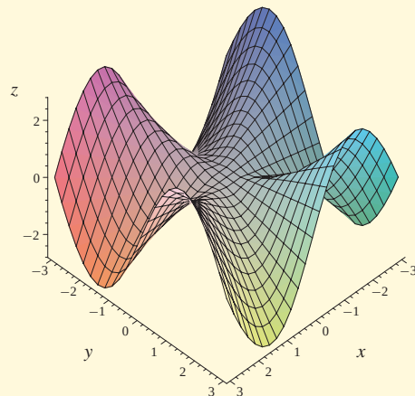
Obr. 2.3: Graf funkce s nezaměnitelnými smíšenými derivacemi v počátku
