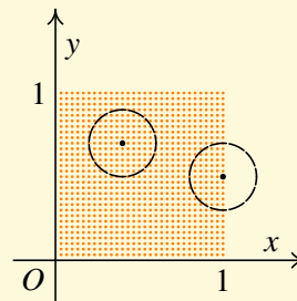
Obr. 1.3: Hranice množiny
