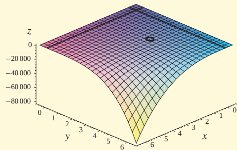
a) (x, y) \in \langle -0,5; 6,5 \rangle \times \langle -0,5; 6,5 \rangle
