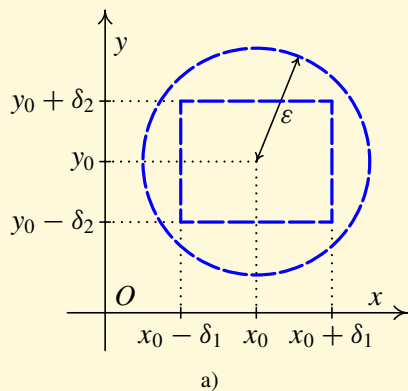
Obr. 1.1: Okolí a klasifikace bodů v rovině
