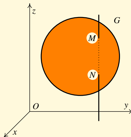
b) G není grafem funkce
