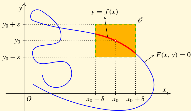
Obr. 7.2: Funkce daná implicitně
