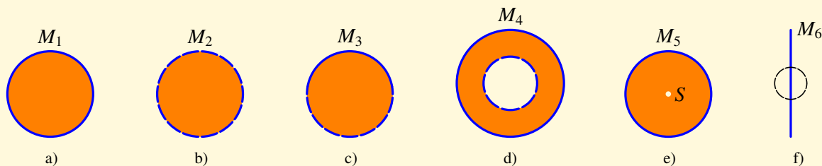
Obr. 1.2: Množiny v rovině
