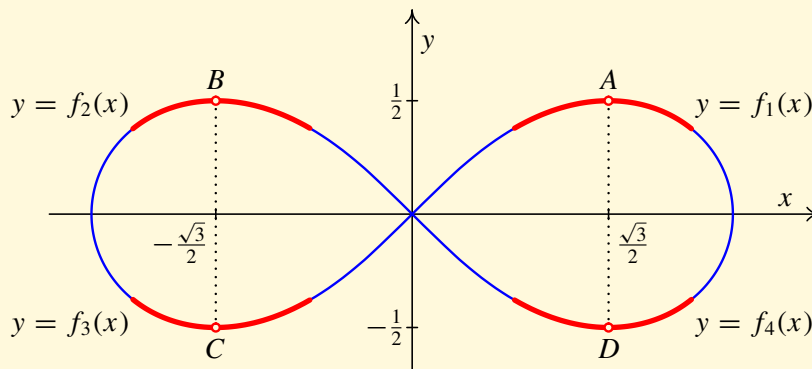
Obr. 7.4: Bernoulliiova lemniskáta
