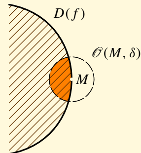
b) Hraniční bod D(f)
