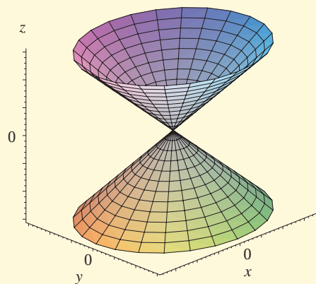
c) Kužel
