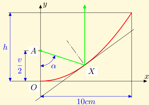
Obr. 7.8: Řez světlometem z příkladu 7.10 Obr. 7.9: Odraz paprsku z příkladu 7.10a)
