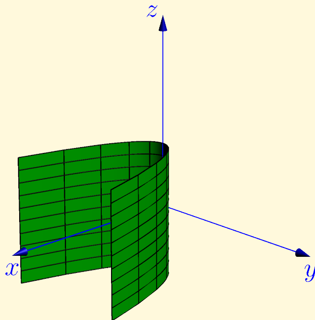
Obr. 8.10: Parabolická válcová plocha((8.16): a = 1 )
