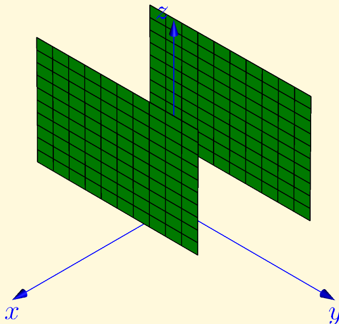
Obr. 8.13: Degenerovaná kvadrika((8.20): c = 1 )
