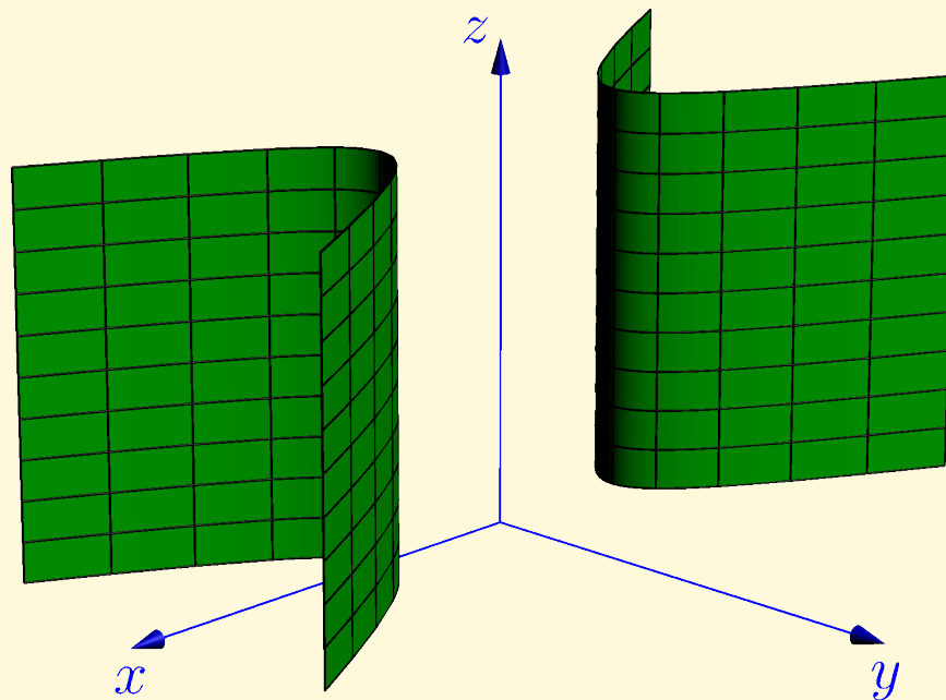
Obr. 8.11: Hyperbolická válcová plocha((8.19): a = 2 , b = 1 )
