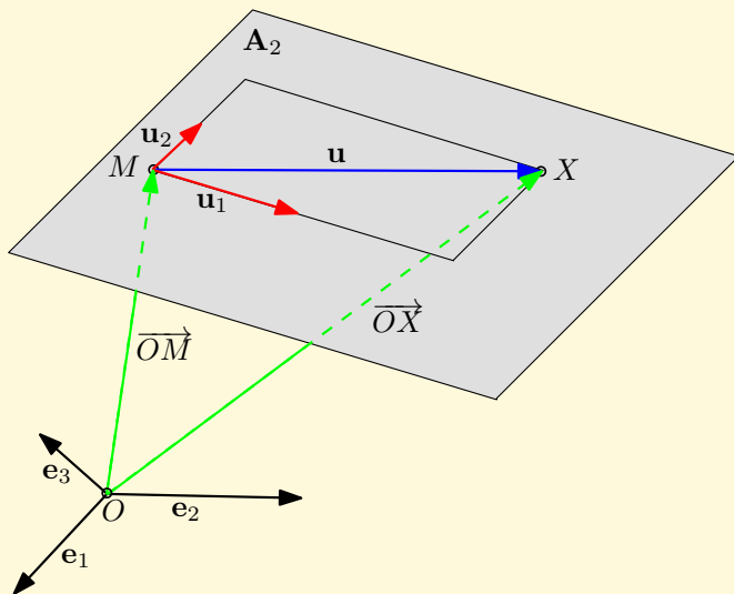
Obr. 2.3: Rovina v afinním prostoru
