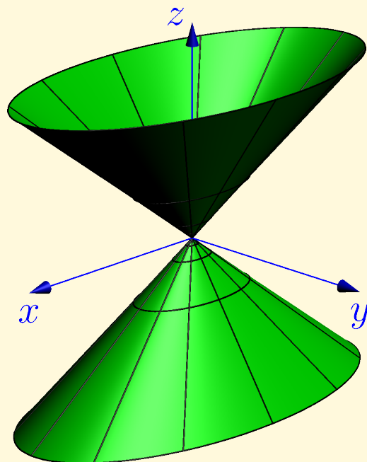
Obr. 8.7: Eliptická kuželová plocha((8.15): a = 4 , b = 2 , c = 1 )
