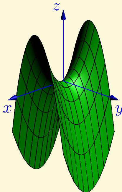
Obr. 8.9: Hyperbolický paraboloid((8.17): a = 2 , b = 1 )
