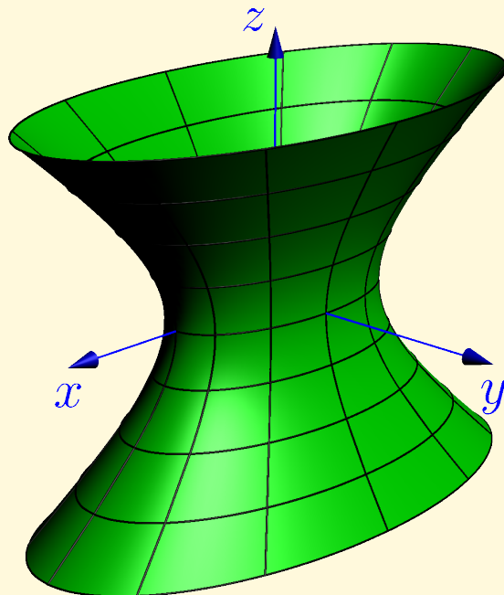
Obr. 8.5: Jednodílný hyperboloid((8.13): a = 4 , b = 2 , c = 1 )
