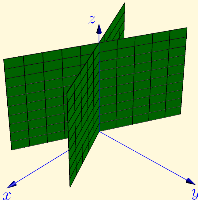
Obr. 8.12: Degenerovaná kvadrika((8.19): a = 2 , b = 1 )
