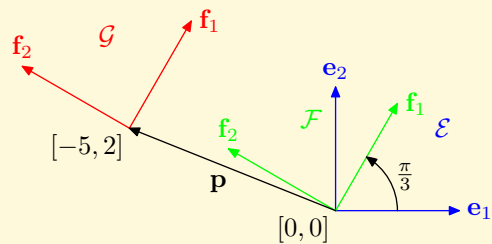
Obr. 7.6: Afinní soustavy souřadnic
