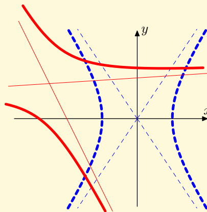
Obr. 7.7: Otočená a posunutá hyperbola
