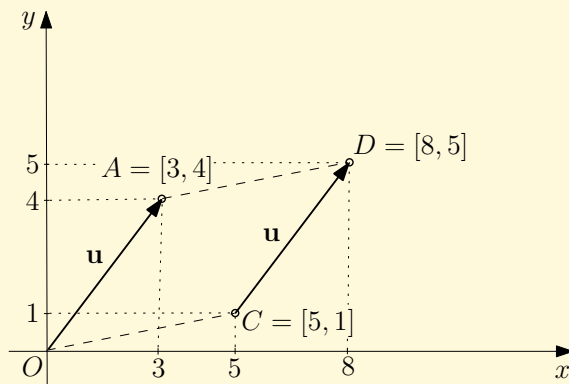
Obr. 1.1: K pojmu vektoru
