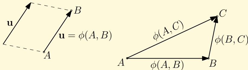
Obr. 2.1: K definici afinního prostoru \mathbf{A}_n
