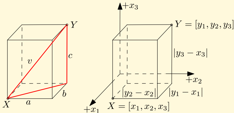
Obr. 3.2: Vzdálenost dvou bodů v \mathbf{E}_3
