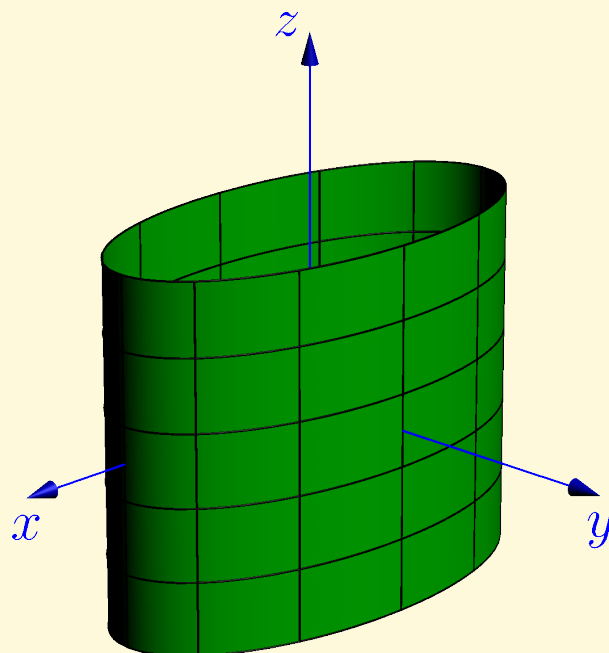
Obr. 8.8: Eliptická válcová plocha((8.16): a = 4 , b = 2 )
