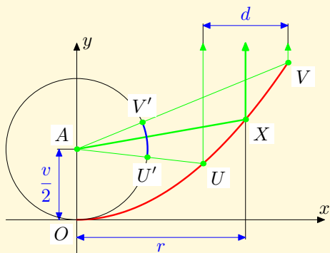
Obr. 7.10: Odraz svazku paprsků
