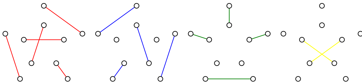
Obrázek 7.4.: Čtyři barvené třídy dobrého hranového barvení Petersenova grafu z Obrázku 7.3.
