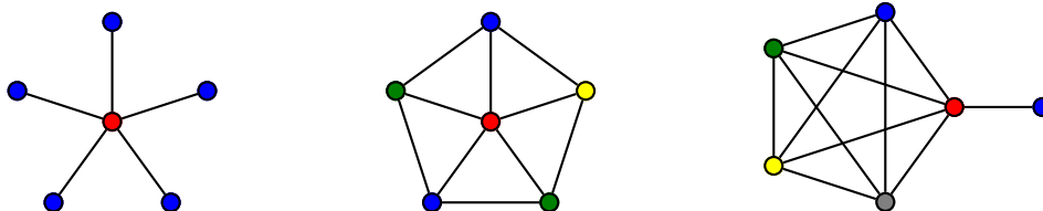
Obrázek 8.1.: Dobré vrcholové barvení hvězdy K_{1,5} , kola W_{1+5} a lízátko L_{5,1} .
