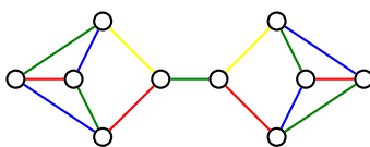
Obrázek 7.8.: Planární graf, který je třídy 2.
