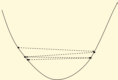
Obr. 4.3: Příliš dlouhý krok
