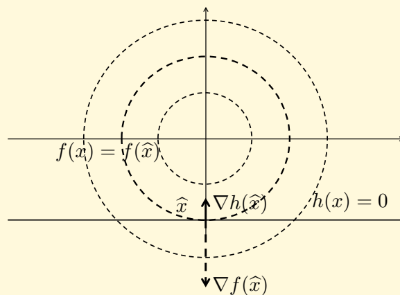
Obr. 9.4: Minimum kvadratické funkce na přípustné množině
