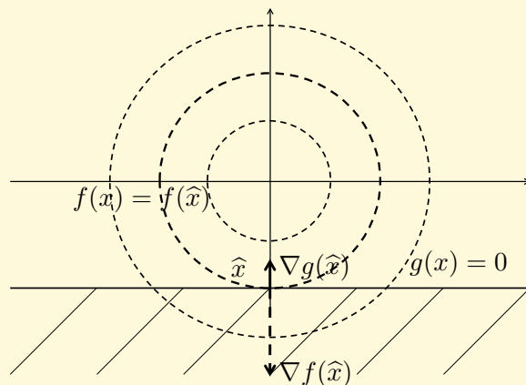
Obr. 11.6: Minimum kvadratické funkce na přípustné množině
