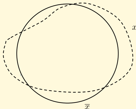
Obr. 1.2: Didonina úloha
