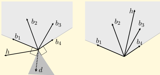
Obr. 11.3: Farkasova věta: řešení úlohy (I) (vlevo) a (II) (vpravo)
