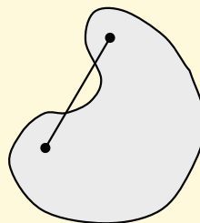
Obr. 2.2: Nekonvexní množina
