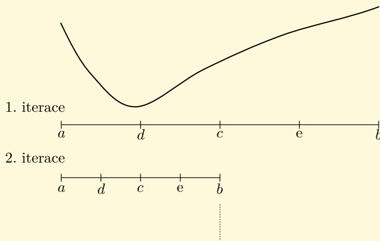
Obr. 3.2: Algoritmus bisekce
