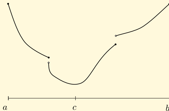
Obr. 3.1: Příklad unimodální funkce
