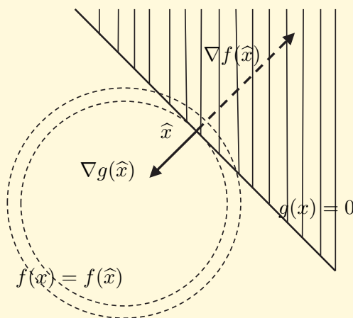
Obr. 11.1: Minimum kvadratické funkce na polovině
