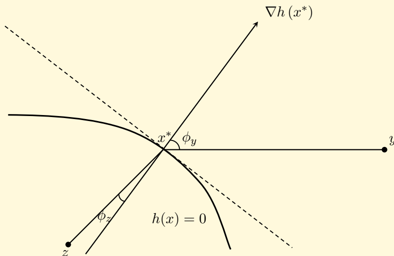
Obr. 9.6: Snellův zákon lomu
