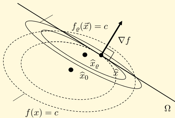
Obr. 10.1: Význam kvadratické penalty
