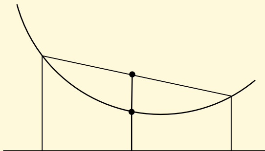
Obr. 2.3: Konvexní funkce
