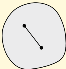
Obr. 2.1: Konvexní množina
