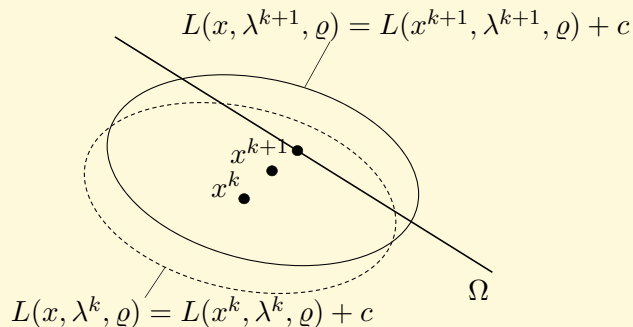
Obr. 10.2: Iterace metody rozšířených Lagrangiánů
