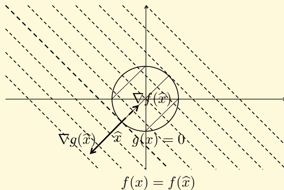
Obr. 11.5: Minimum lineární funkce na přípustné množině
