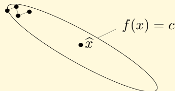
Obr. 4.2: Pomalá konvergence metody největšího spádu
