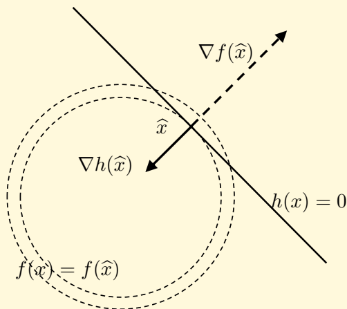
Obr. 9.1: Minimum kvadratické funkce na přímce
