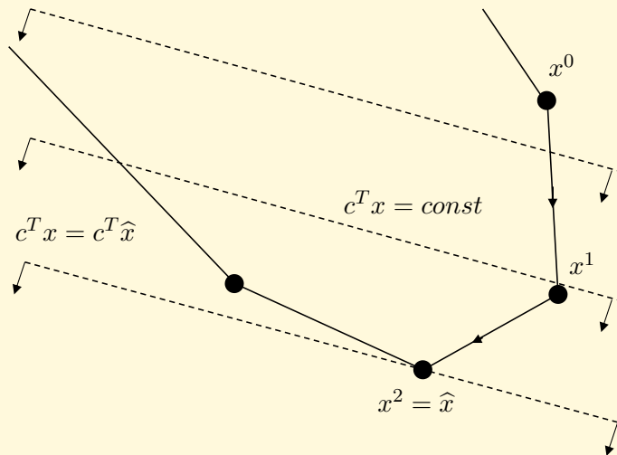
Obr. 14.1 Geometrické znázornění simplexové metody
