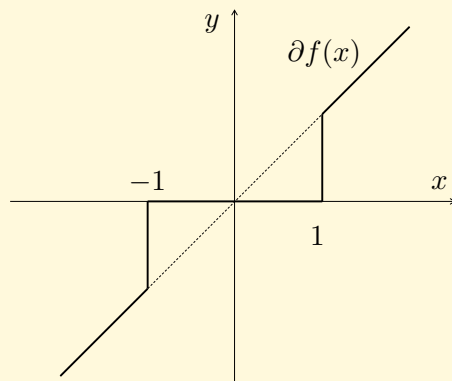
Obr. 15.4: Zobecněný gradient \partial f(x) funkce f(x) = \max \{0, \frac{1}{2} (x^2 - 1)\}
