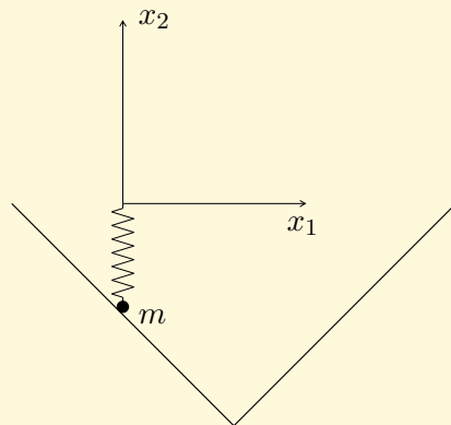
Obr. 1.1: Rovnovážný stav kuličky na pružině
