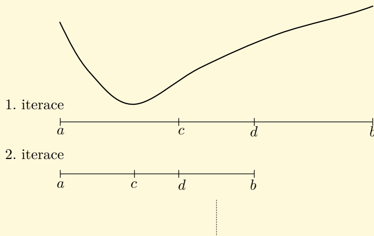
Obr. 3.4: Algoritmus zlatého řezu
