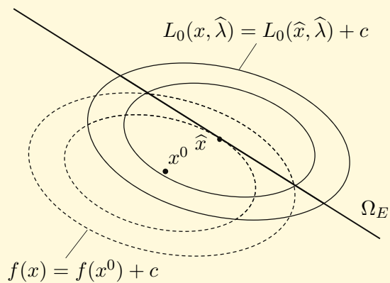
Obr. 9.2: Geometrický význam Lagrangianu
