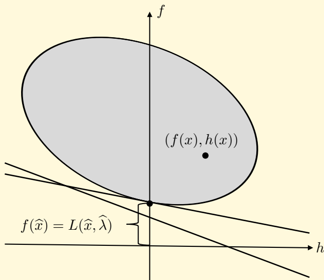
Obr. 13.1: Ilustrace vizualizačního lematu
